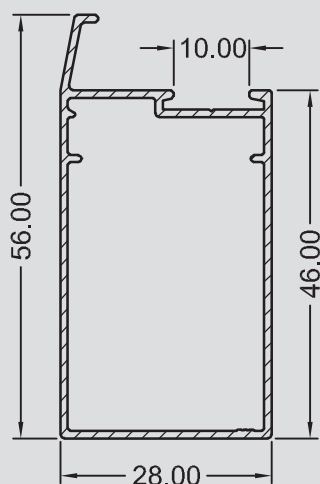
P-0530 0,452 kg/m
