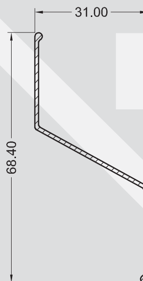
SP - 0455 0,255 kg/m
