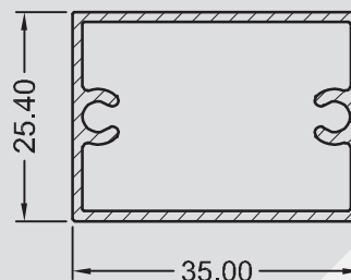
D - 0055 0,457 kg/m
