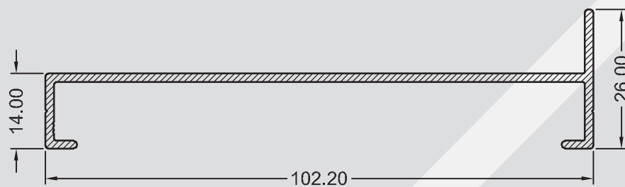
LG-0002 0,633 kg/m
