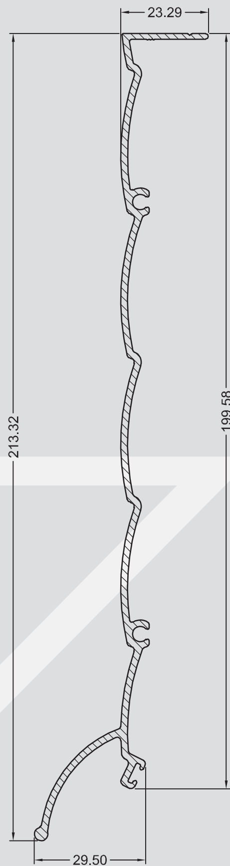
MN-0039 1,396 kg/m
