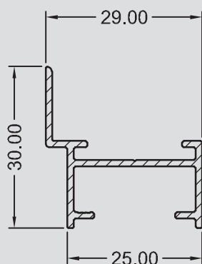
SU-0071 0,275 kg/m
