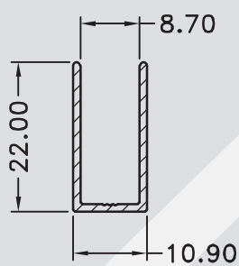
U - 0606 0,154 kg/m
