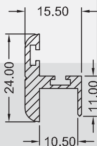
Y - 0343 0,307 KG/M
