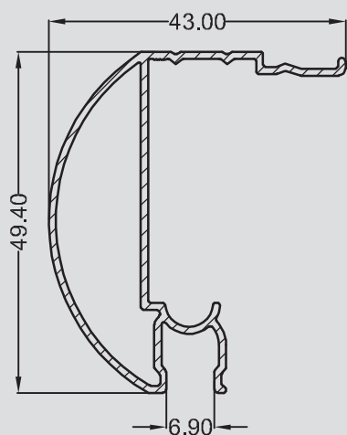
SP - 0446 0,482 KG/M
