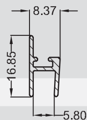
SP - 0451 0,104 KG/M
