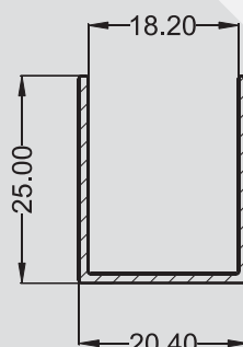
SP - 0121 0,203 kg/m
