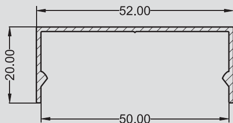
U - 0877 0,335 kg/m
