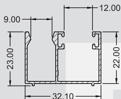
SP-0647 0.315 KG/M
