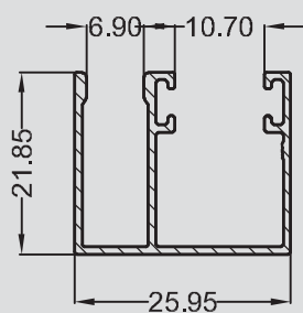
SP - 0448 0,259 KG/M
