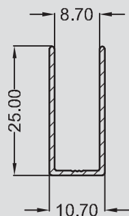
SP - 2154 0,156 KG/M
