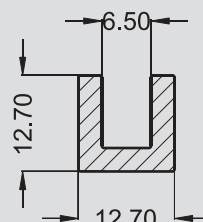
U - 0306 0,267 kg/m
