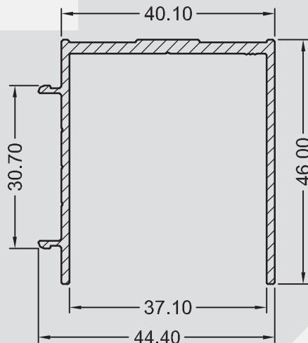
SP - 0593 0,636 KG/M
