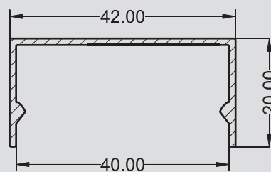
U - 0621 0,293 kg/m
