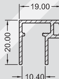
SP - 0967 0,239 KG/M
