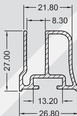
SP - 0594 0,456 KG/M
