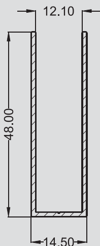
SP - 0122 0,350 kg/m
