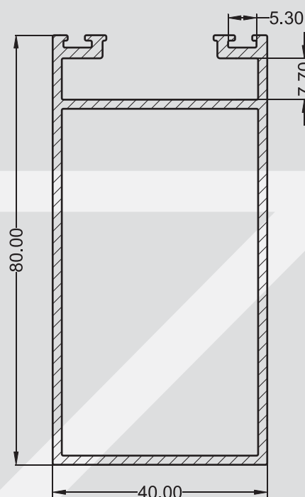
A - 0072 1,200 kg/m
