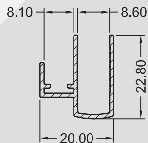
SP - 0589 0,214 kg/m
