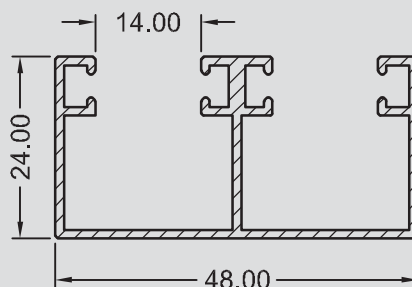
SP - 0277 0,510 KG/M
