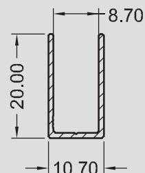
SP - 0474 0,130 KG/M
