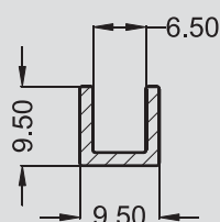
U - 0036 0,106 kg/m
