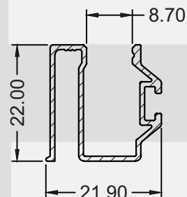
SP-0574 0.238 KG/M
