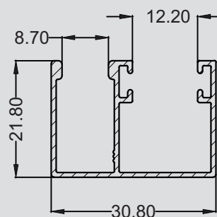
SP-0551 0.286 KG/M
