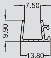
SP-0552 0.099 KG/M
