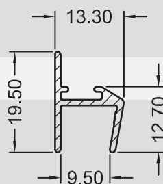
SP - 0559 0,142 KG/M
