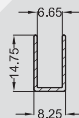
SP - 0453 0,079 KG/M
