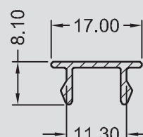
U - 0491 0,105 KG/M
