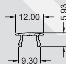
SP - 0217 0.053 KG/M
