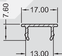
SP - 0547 0,088 KG/M
