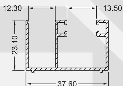
E - 0306 0,375 KG/M
