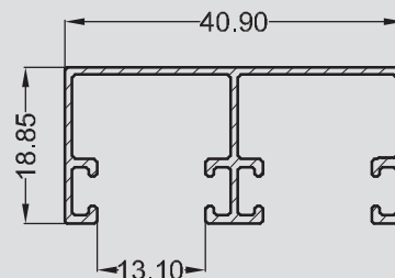
SP-0433 0,320 kg/m
