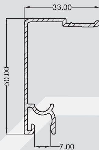
SP - 0560 0,432 KG/M
