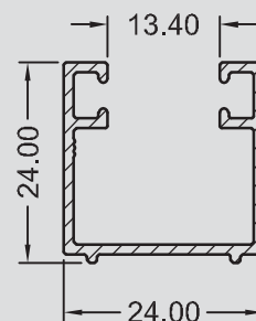
U - 1108 0,293 KG/M
