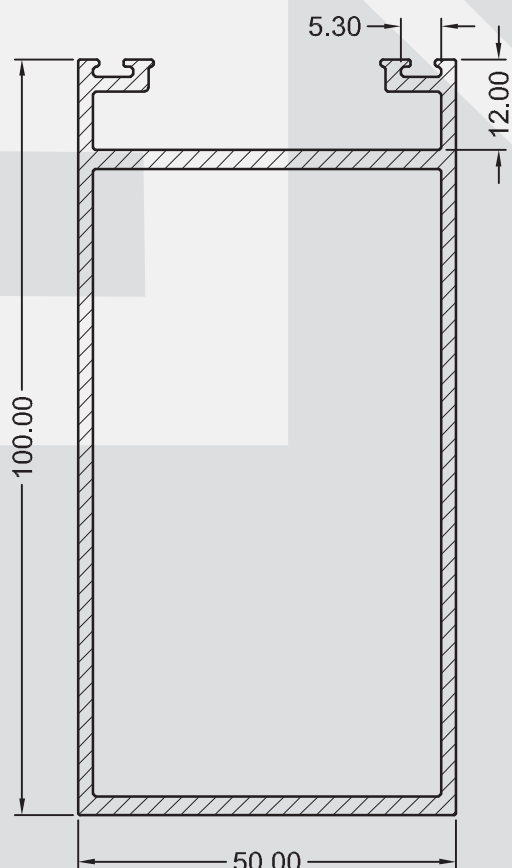
A - 0096 1,847 kg/m
