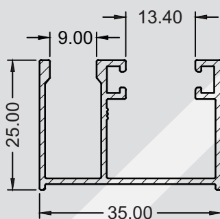
SP-0565 0.391 KG/M
