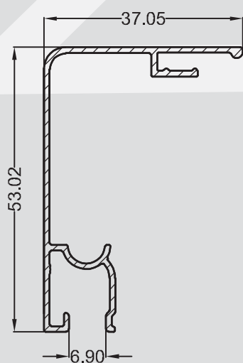
SP - 0447 0,414 KG/M
