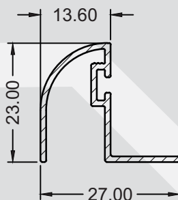
SP-2297 0.220 KG/M
