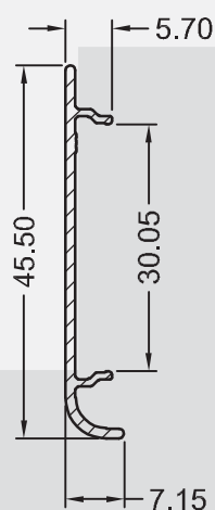
SP - 0596 0,187 KG/M
