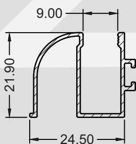
SP-0724 0.233 KG/M
