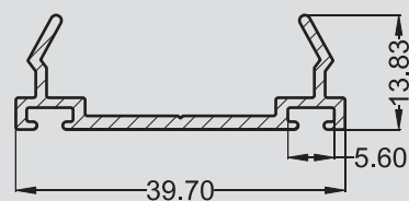
U - 0615 0,285 kg/m
