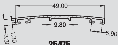
25475 0,233 kg/m
