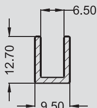
U - 0037 0,135 kg/m
