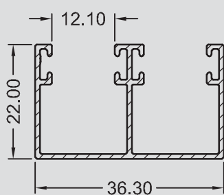
SP - 2969 0,318 KG/M
